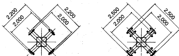
■台座平面図 (単位: mm)
