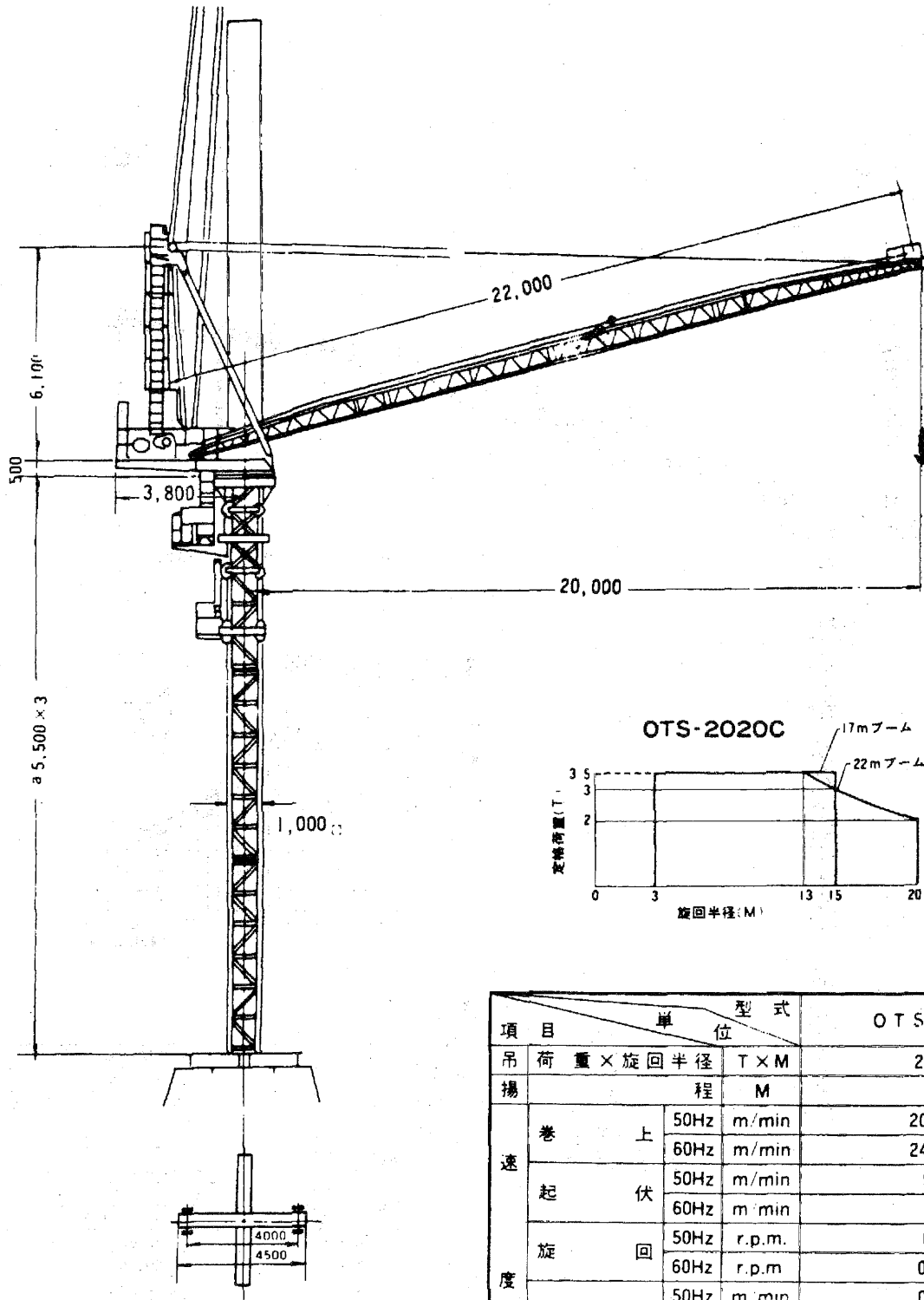
OTS-2020C型
